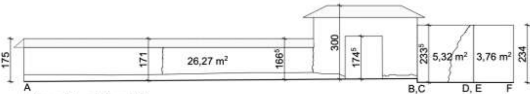
Elevation Mur 25
